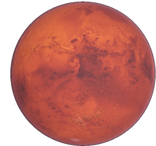
Mars
