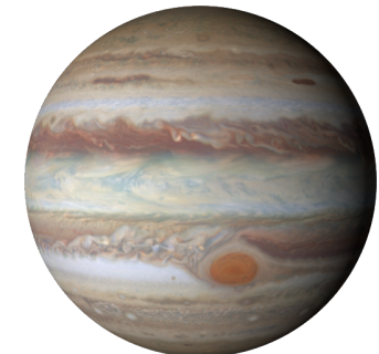
Jupiter
