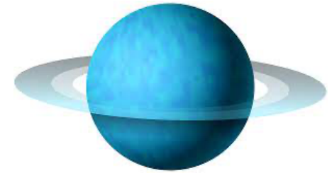
Uranus
