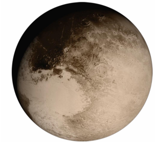
Pluto
