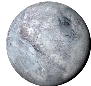
Eris
