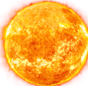
Sun
