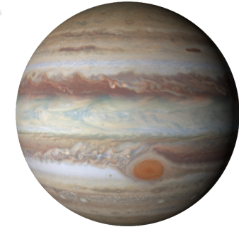
Jupiter
