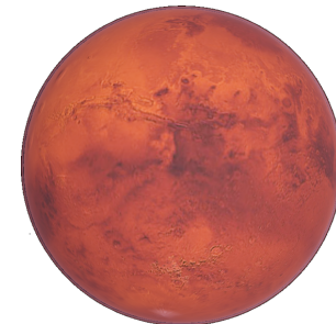
Mars
